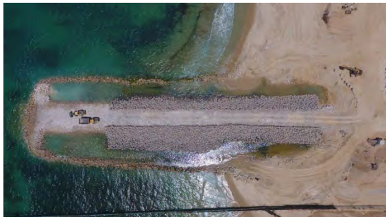
בניית המכשול הימי סמוך לחוף זיקים (דוברות משרד הביטחון, 5 באוגוסט 2018)
