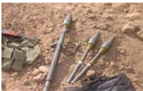
רקטות מסוג "אליאסין" תוצרת החמא"ס טווח מקסימלי: כ-250 מ' כושר חדירה משוער: עד 200 מ"מ פלדה
